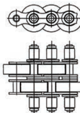
D Duplex mit versetzten Stauförderrollen Duplex with offset accumulation rollers
